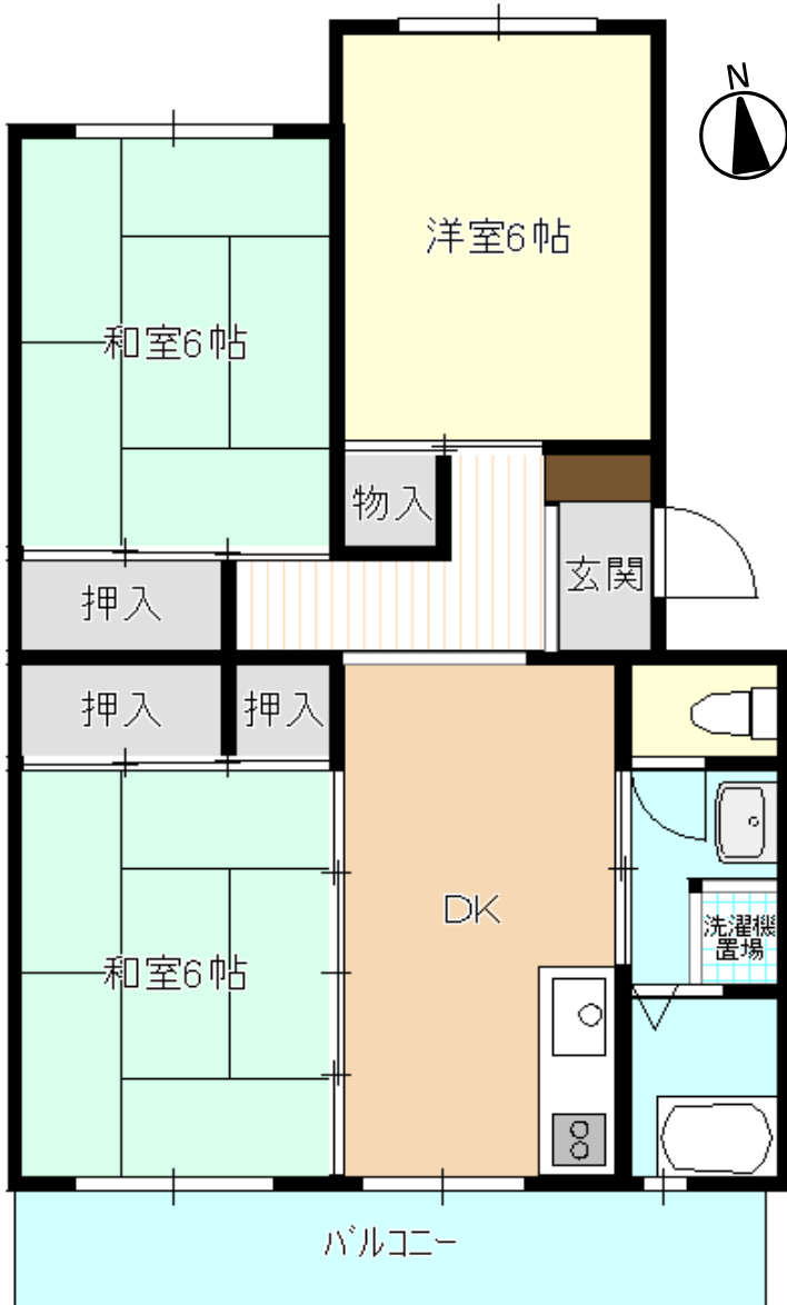
《間取り図》
