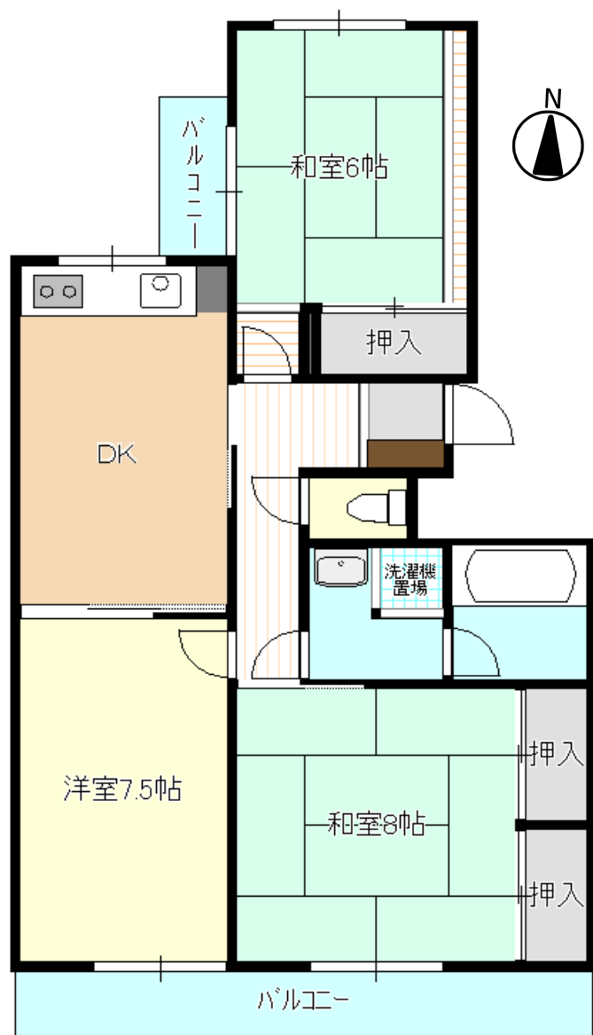
《間取り図》
