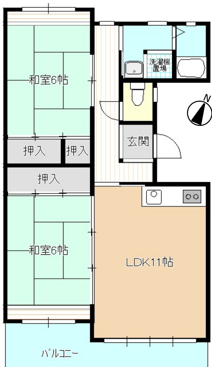
《間取り図》
